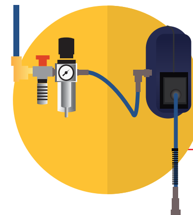
LÍNEA DE AIRE PARA LIMPIEZA DE CILINDROS
